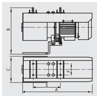
Тельфер
