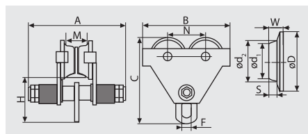
Каретка для тали
