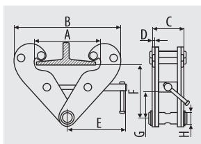
Каретка для тали
