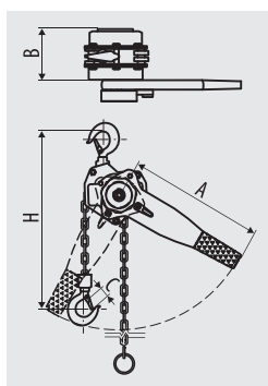
Таль рычажная
