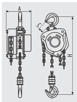
Таль цепная стационарная
