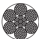
6x37 + IW RC
